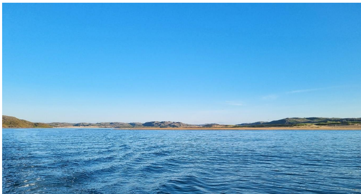
Рис 6. Долина реки Воронья близ устья. Песчаные дюны
